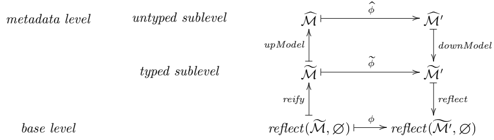
Figure 5.1: M2 sublevels.
